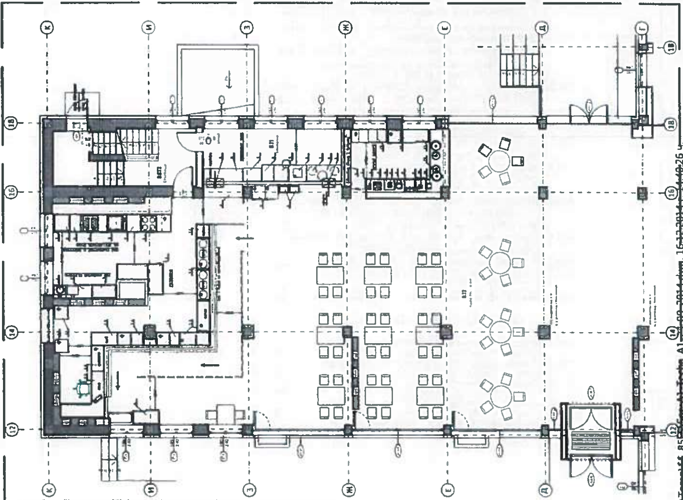
ПРИЗЕМЕН ЭТАЖ / GROUND FLOOR
